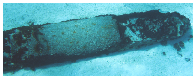
Um torpedo limpo (em cima) e outro altamente corroído no fundo do mar (em baixo).
